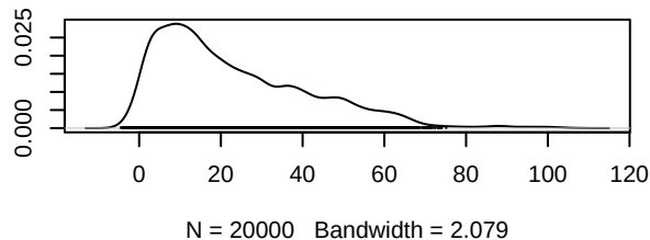
Density of d.Gefitinib.Gefitinib_PARPi
