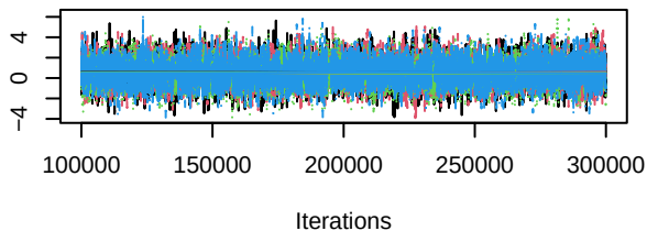
Trace of d.Erlotinib.Rociletinib
