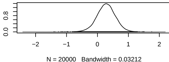
Density of d.Erlotinib.Erlotinib_antiangio
