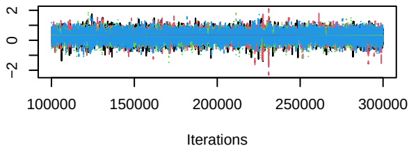
Trace of d.Erlotinib.Erlotinib_antiangio
