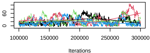
Trace of d.Gefitinib.Gefitinib_PARPi
